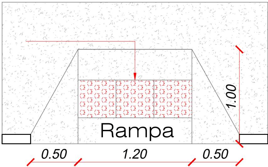
Detalhe Rampa PNE Esc. 1:50
