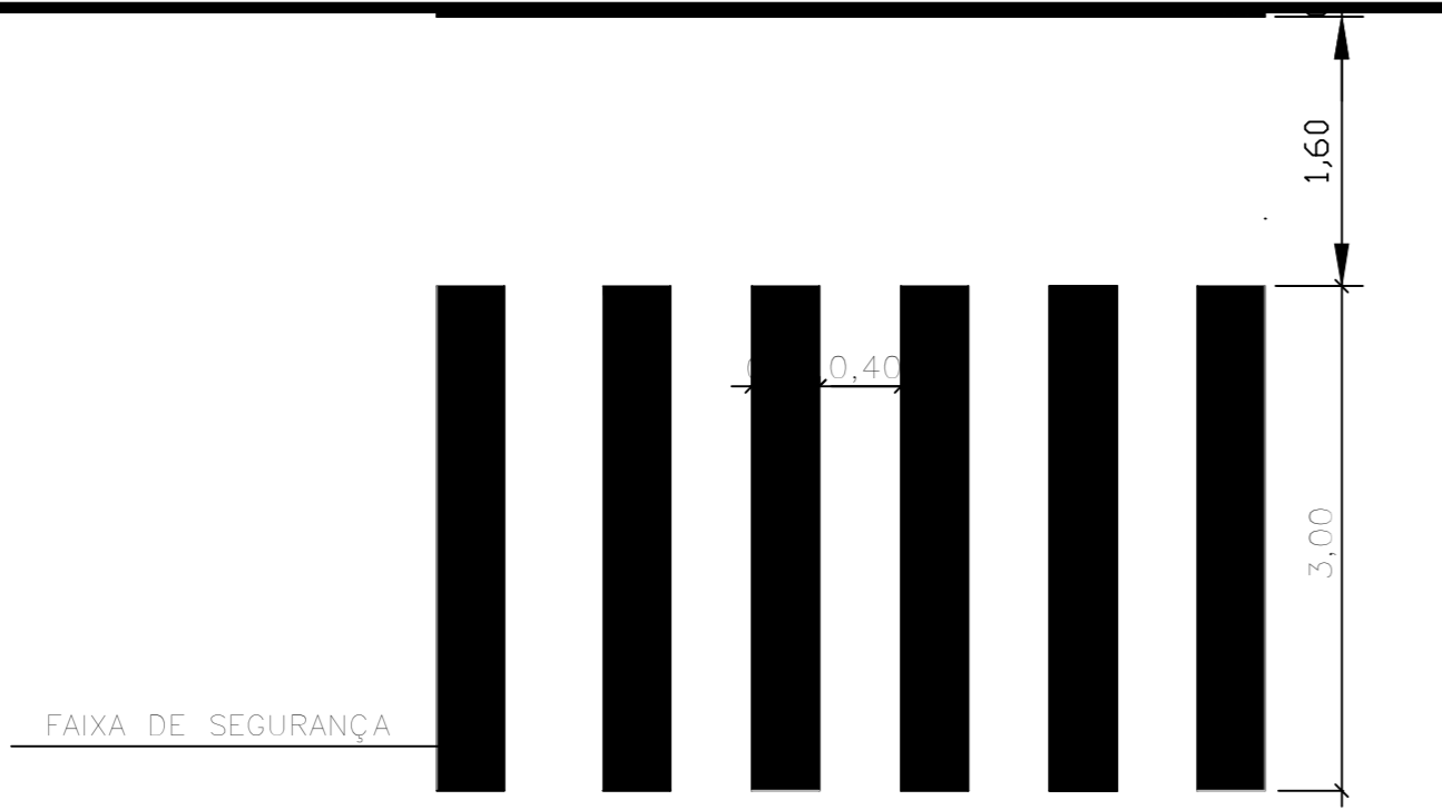
DETALHE 01 FAIXA DE SEGURANÇA Sem escala Tinta: EXTRUDADO Cor: BRANCA
