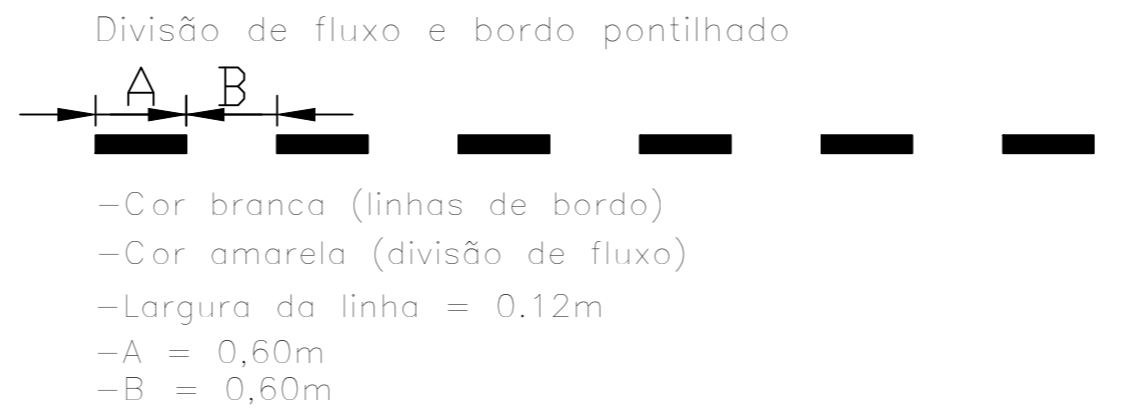
DETALHE 02 Divisão de fluxo e bordo pontilhado Sem escala -Cor branca (linhas de bordo) -Cor amarela (divisão de fluxo) -Largura da linha = 0,12m -A = 0,60m -B = 0,60m
