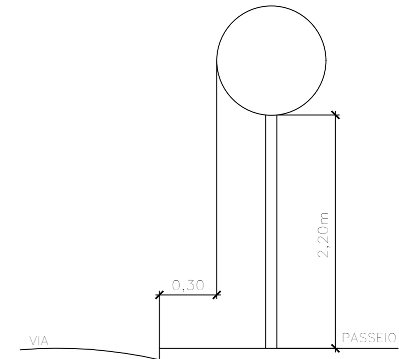
DETALHE 04 LOCAÇÃO DE PLACAS DE SINALIZAÇÃO Sem escala
