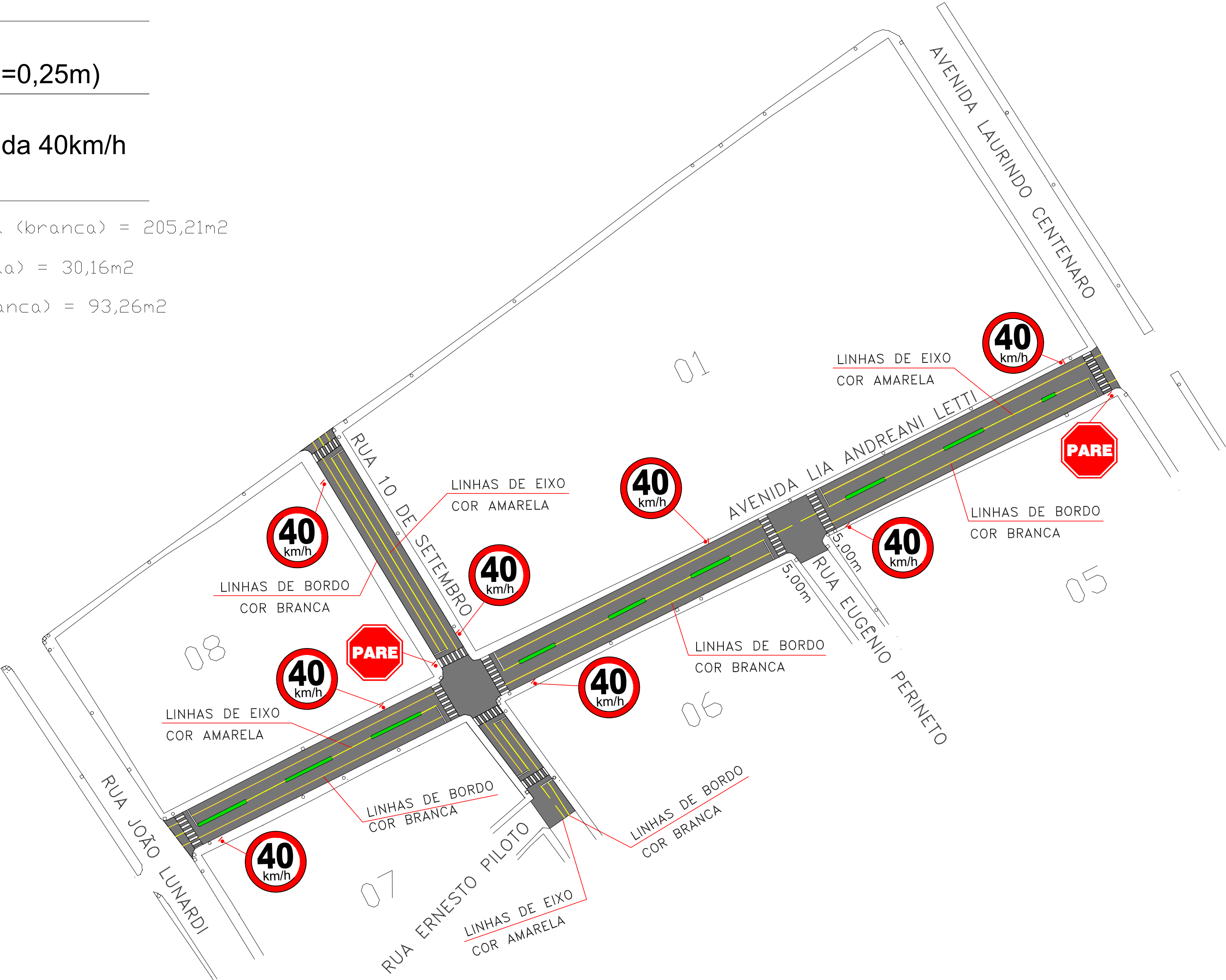
PLANTA SINALIZAÇÃO ESCALA 1:1.000
