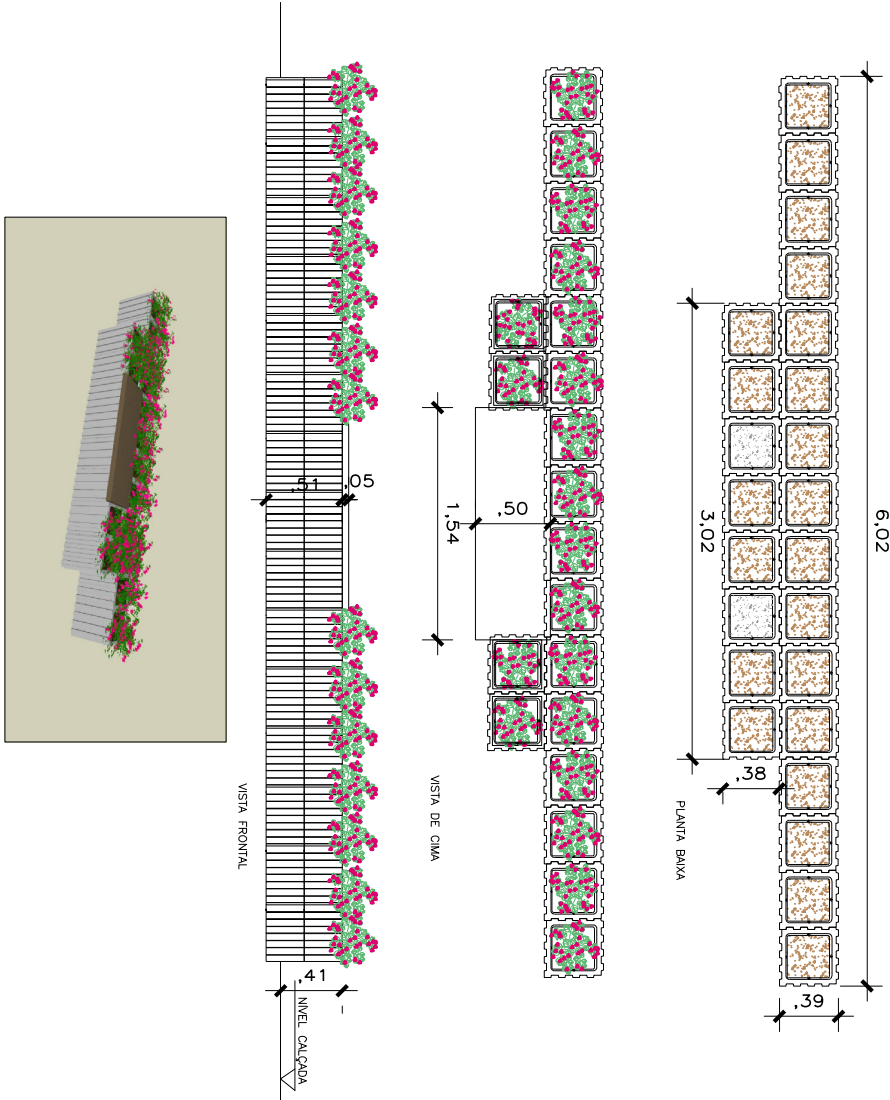
BANCO FLOREIRA – TIPO 1 Esc: 1/50
