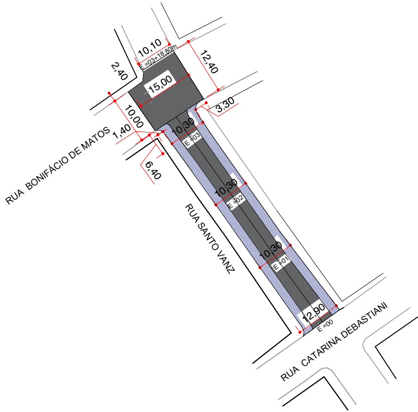
PLANTA PAVIMENTAÇÃO ASFÁLTICA EM CBUQ ESCALA 1:1.000
