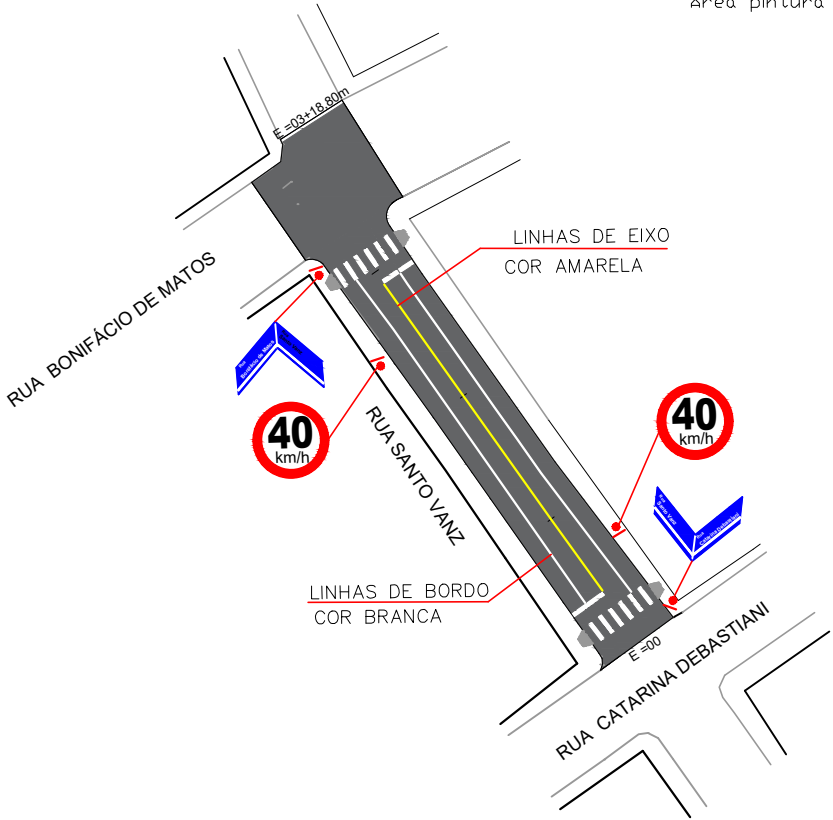
PLANTA SINALIZAÇÃO ESCALA 1:1.000
