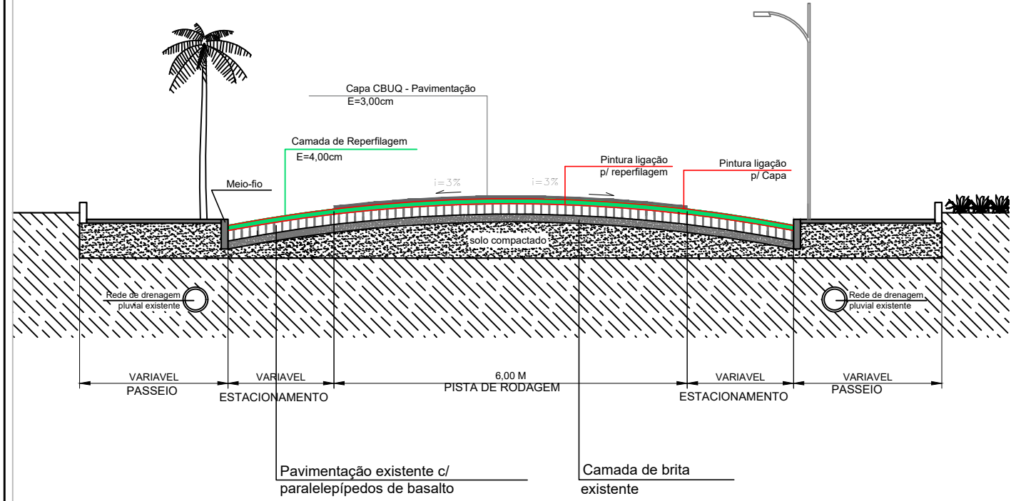
PERFIL VIÁRIO (SEM ESCALA) TRECHO RUA PEDRO LUIZ GRASSI
