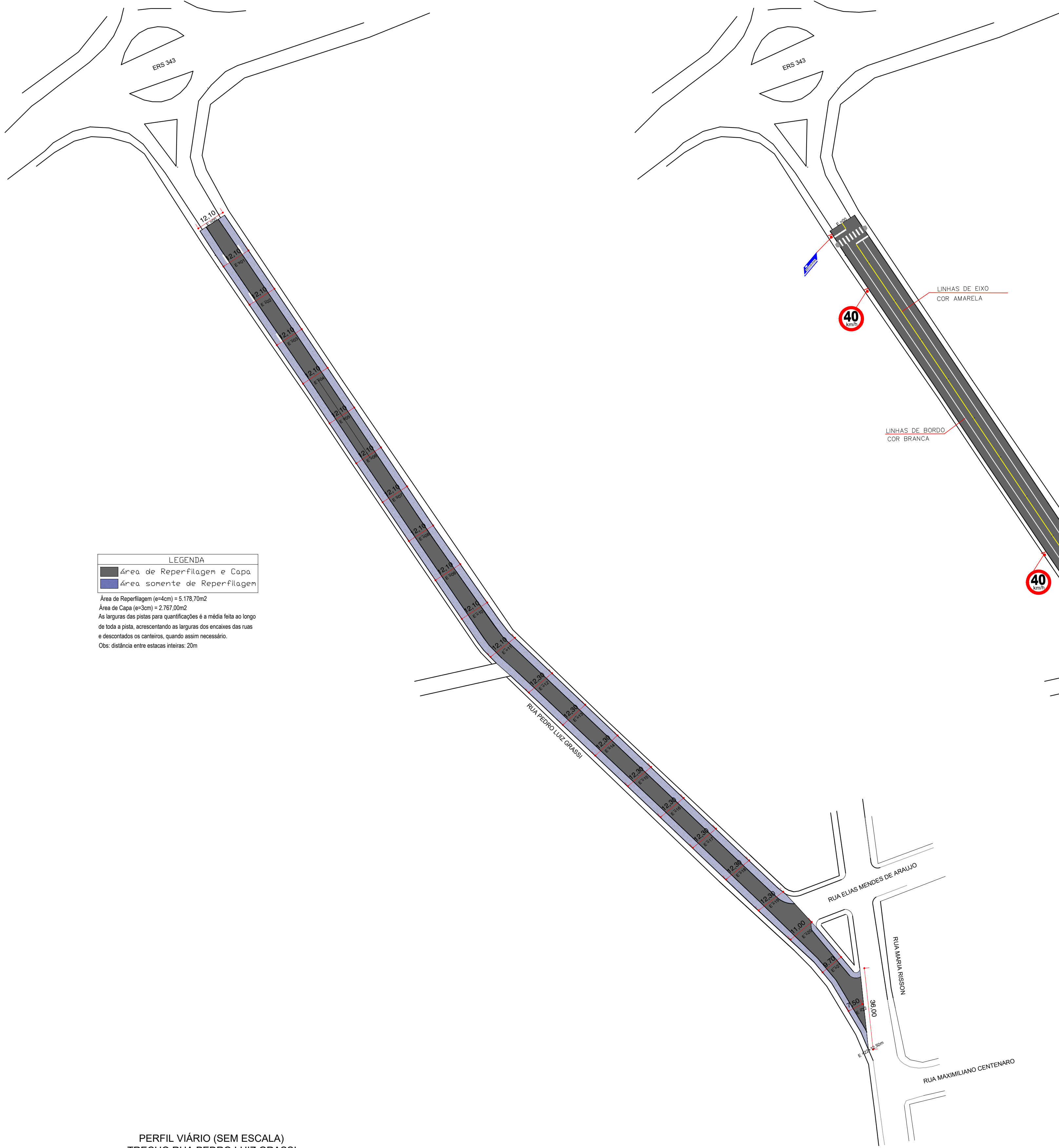
PLANTA PAVIMENTAÇÃO ASFÁLTICA EM CBUQ ESCALA 1:1.000
