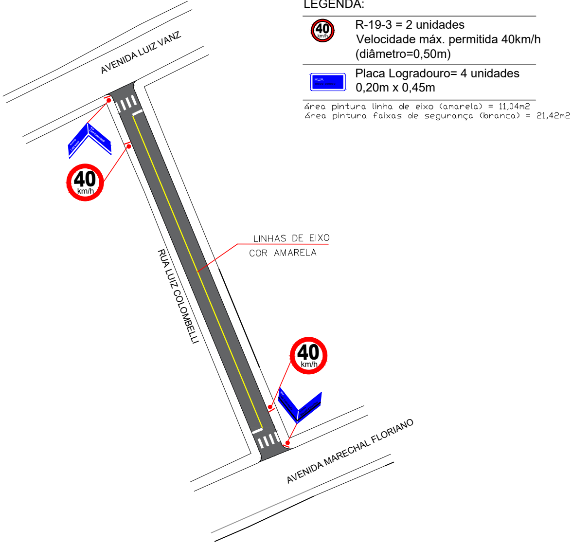
PLANTA SINALIZAÇÃO ESCALA 1:1.000
