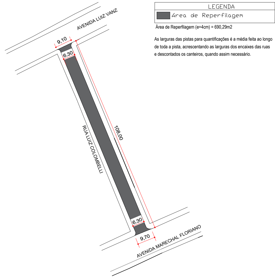
PLANTA PAVIMENTAÇÃO ASFÁLTICA EM CBUQ ESCALA 1:1.000
