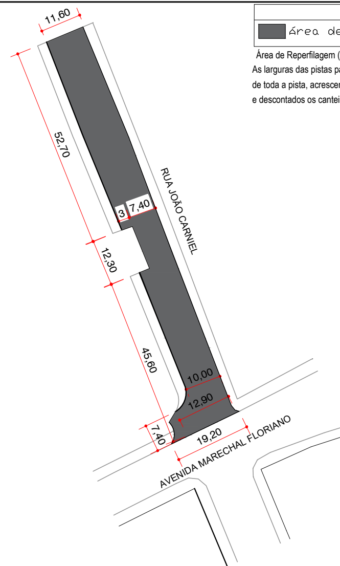
PLANTA PAVIMENTAÇÃO ASFÁLTICA EM CBUQ ESCALA 1:1.000
