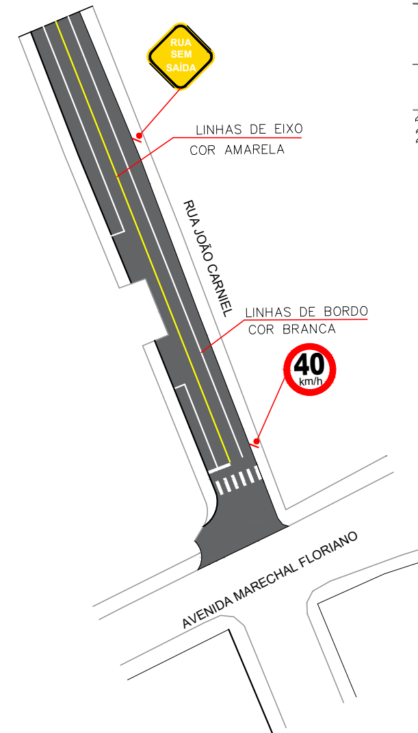
PLANTA SINALIZAÇÃO ESCALA 1:1.000
