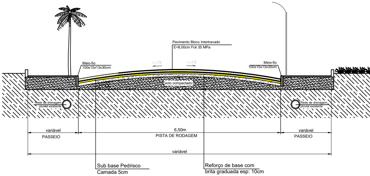
PERFIL VIÁRIO (SEM ESCALA) TRECHO DA RUA PEDRO LOTTICI
