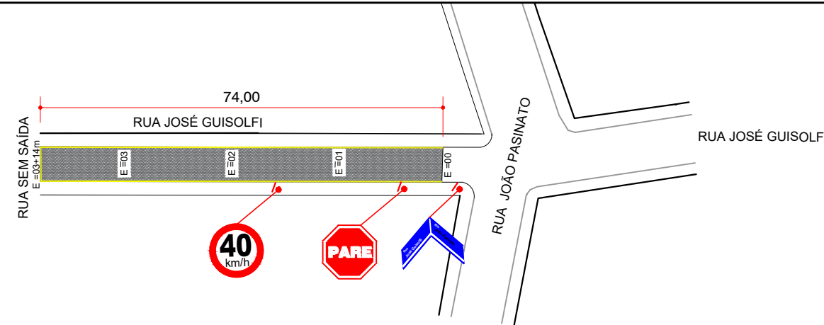
PLANTA PAVIMENTAÇÃO E SINALIZAÇÃO EM BLOCO INTERTRAVADO ESCALA 1:1.000
