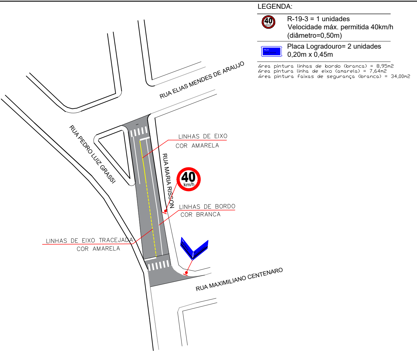
PLANTA SINALIZAÇÃO ESCALA 1:1.000
