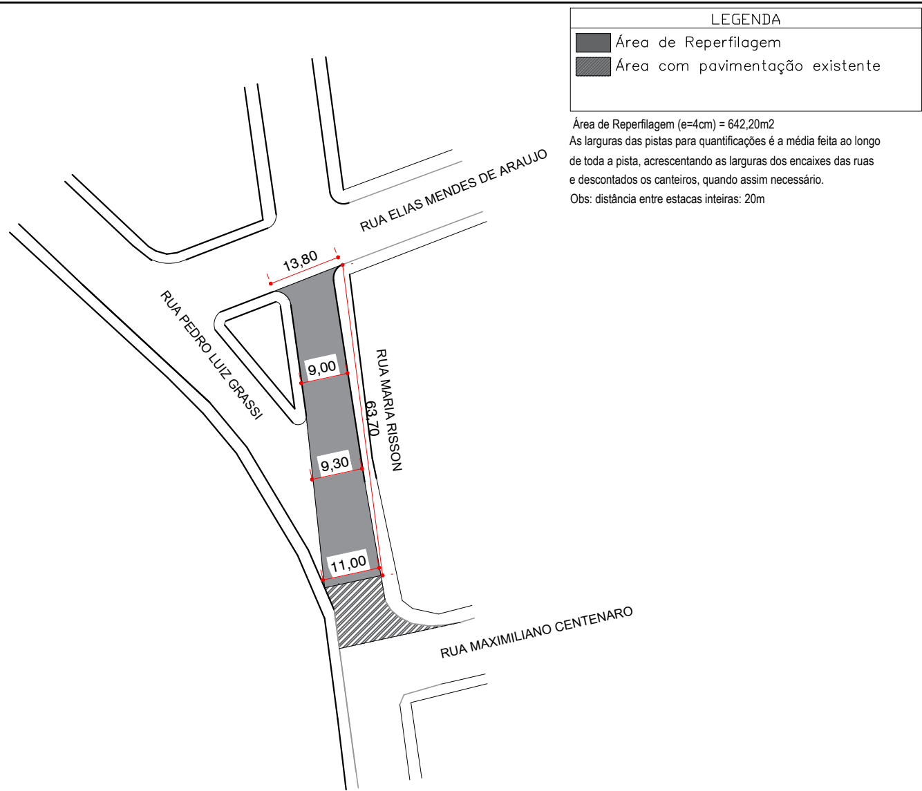
PLANTA PAVIMENTAÇÃO ASFÁLTICA EM CBUQ ESCALA 1:1.000
