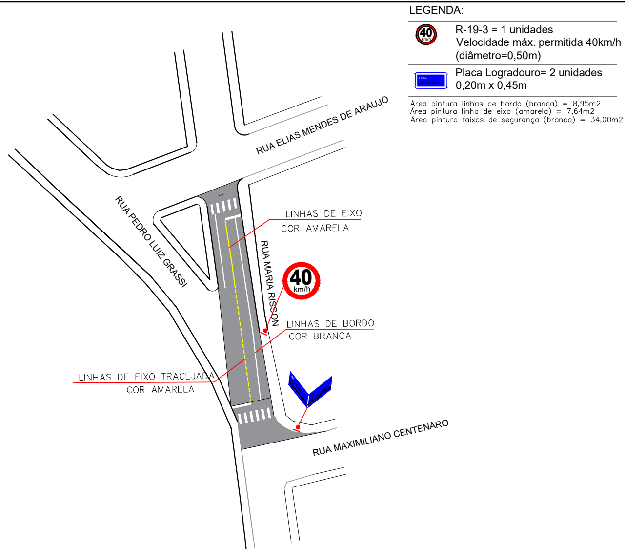
PLANTA SINALIZAÇÃO ESCALA 1:1.000
