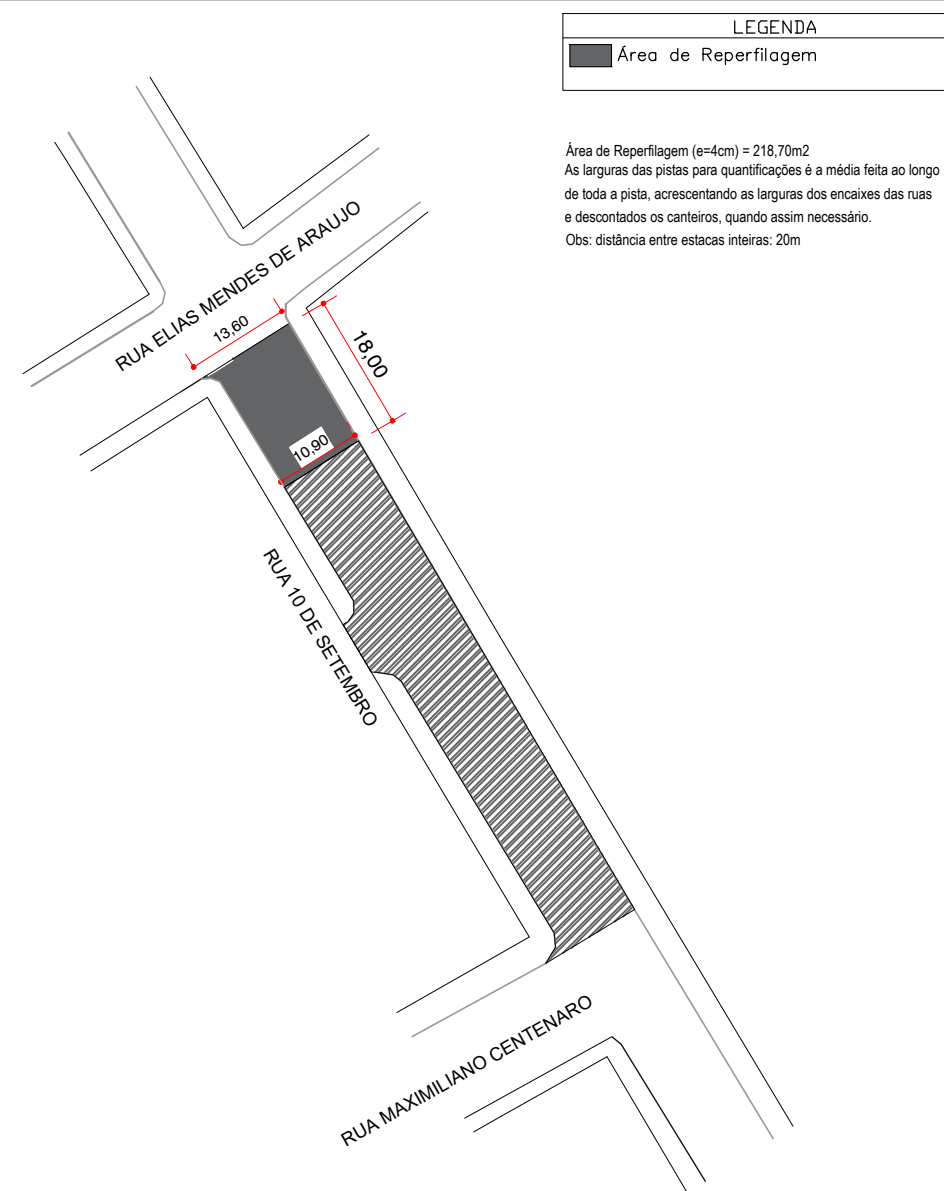
PLANTA PAVIMENTAÇÃO ASFÁLTICA ESCALA 1:1.000
