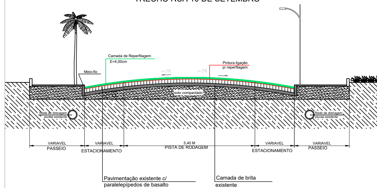
PERFIL VIÁRIO (SEM ESCALA) TRECHO RUA 10 DE SETEMBRO
