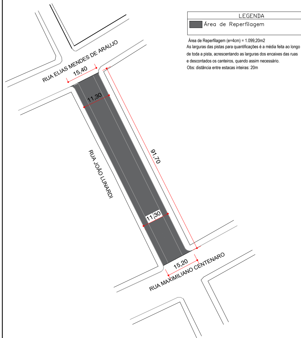
PLANTA PAVIMENTAÇÃO ASFÁLTICA ESCALA 1:1.000
