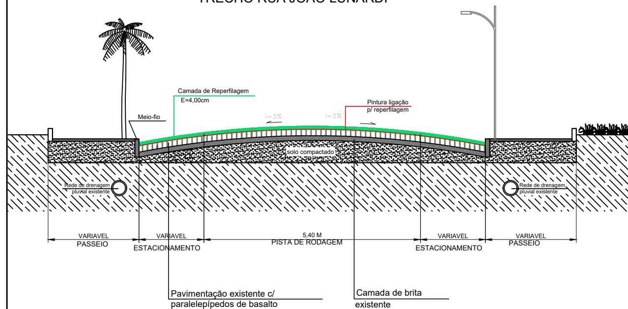
PERFIL VIÁRIO (SEM ESCALA) TRECHO RUA JOÃO LUNARDI
