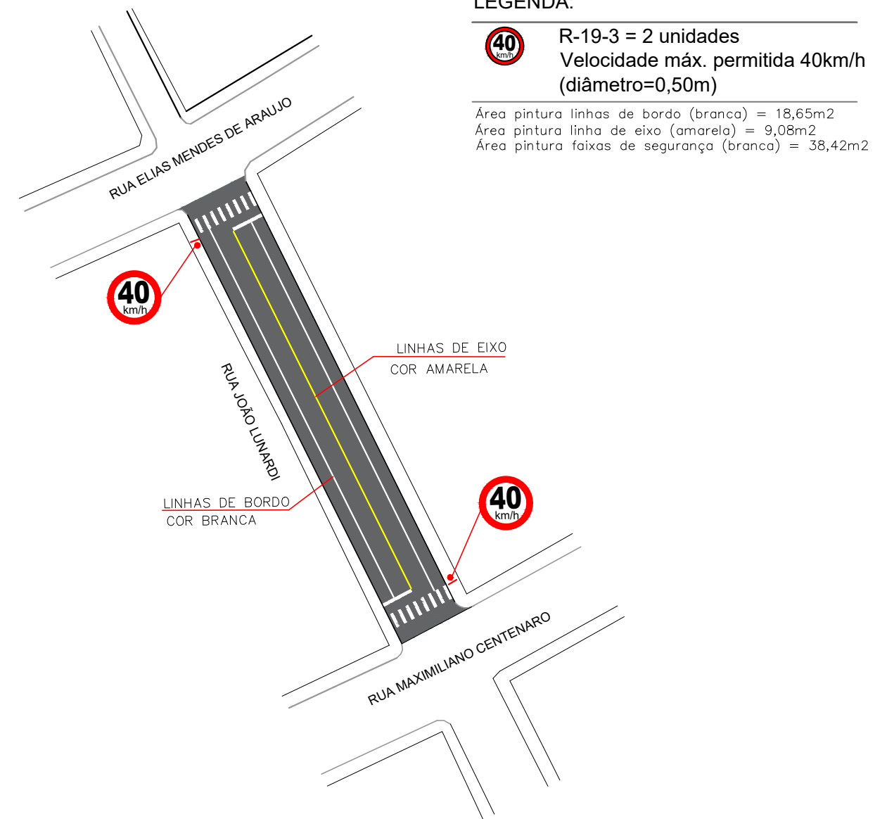
PLANTA SINALIZAÇÃO ESCALA 1:1.000
