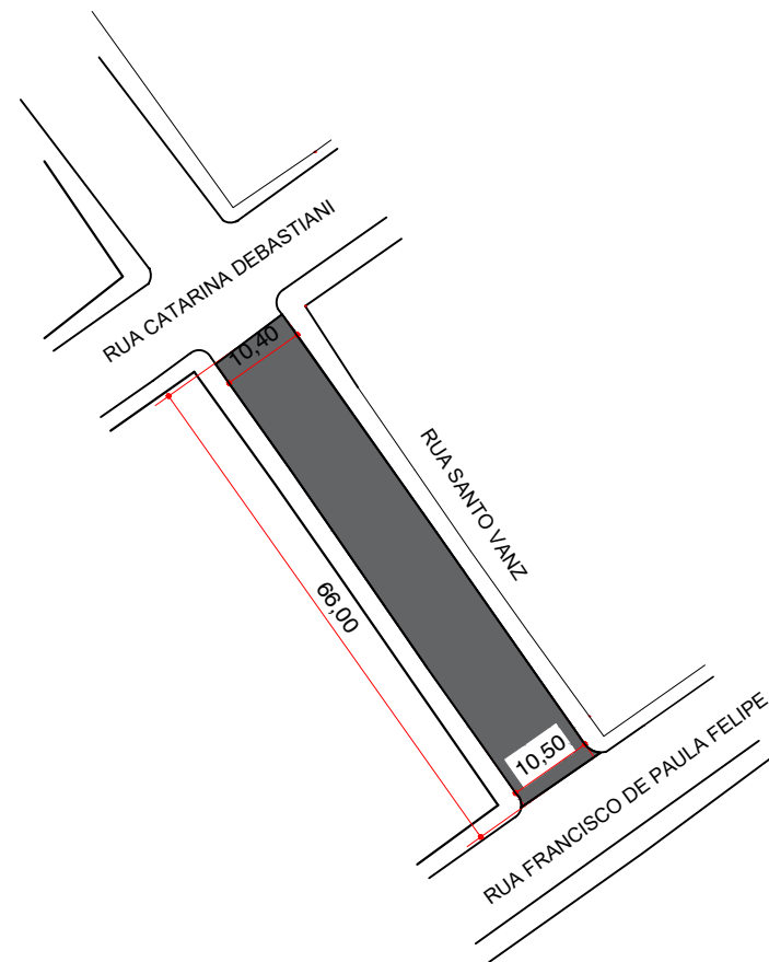
PLANTA PAVIMENTAÇÃO ASFÁLTICA EM CBUQ ESCALA 1:1.000
