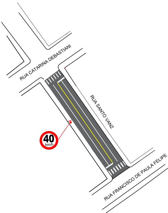
PLANTA SINALIZAÇÃO ESCALA 1:1.000
