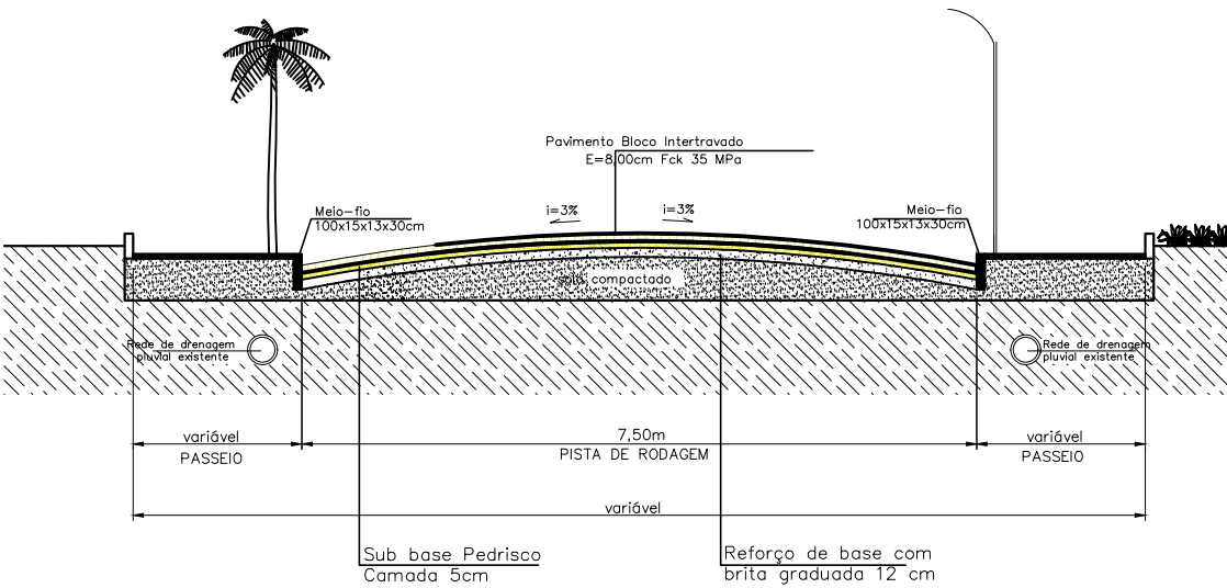
PERFIL VIÁRIO (SEM ESCALA) TRECHO DA RUA ANTONIO FERRARI
