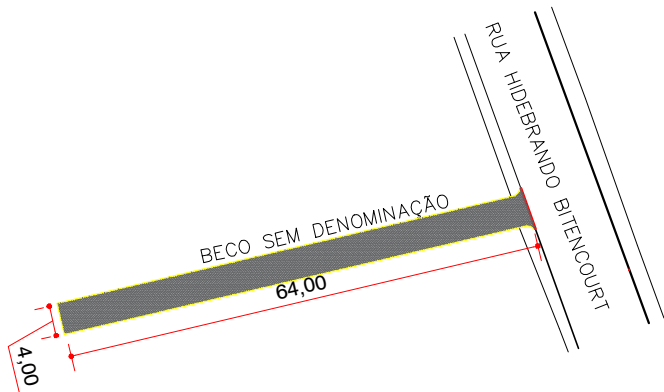
PLANTA PAVIMENTAÇÃO EM BLOCO INTERTRAVADO ESCALA 1:1.000
