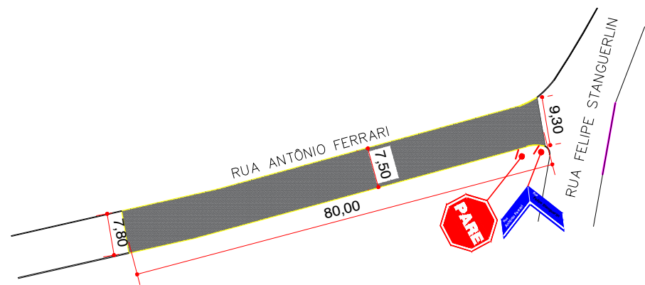
PLANTA PAVIMENTAÇÃO EM BLOCO INTERTRAVADO ESCALA 1:1.000
