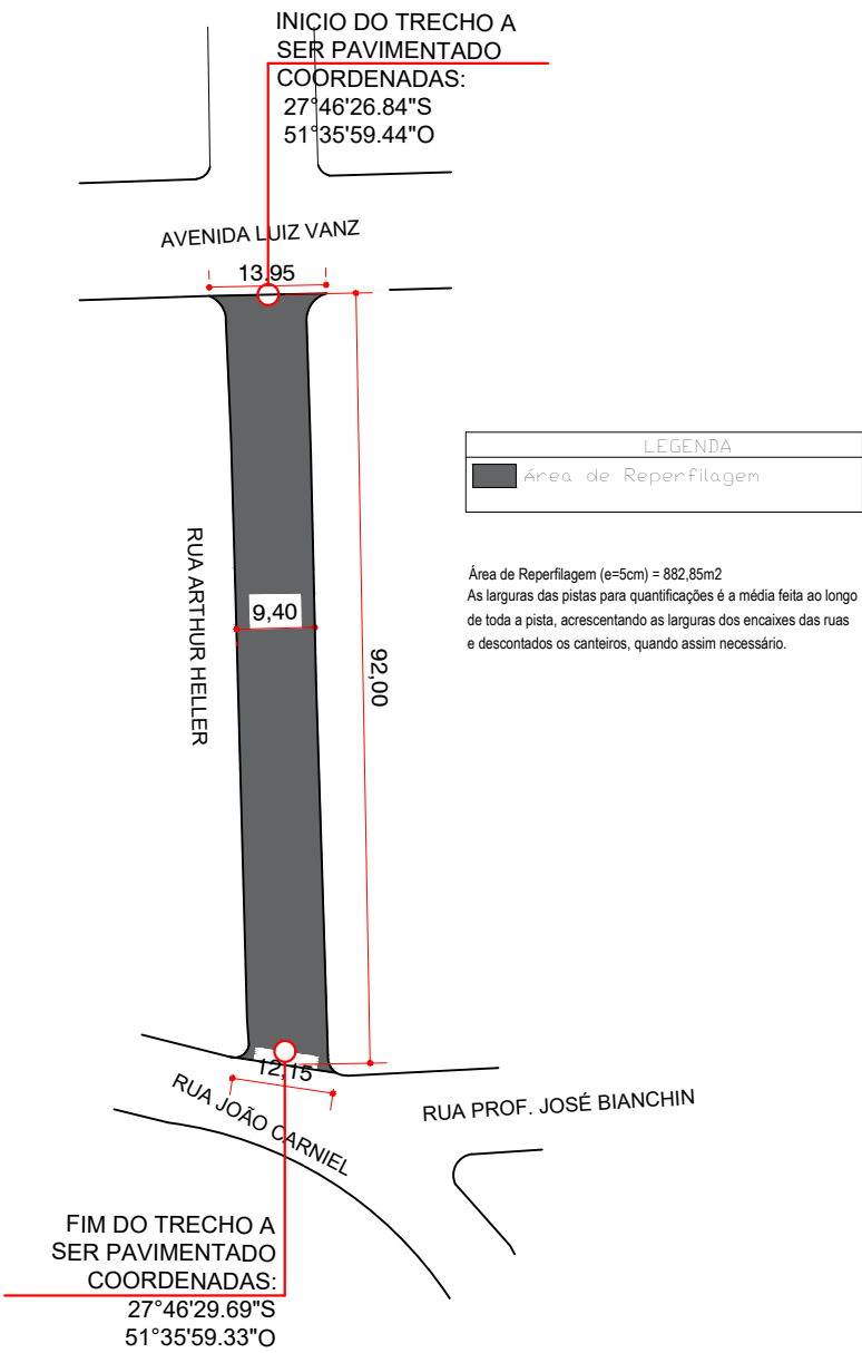
PLANTA PAVIMENTAÇÃO ASFÁLTICA EM CBUQ ESCALA 1:1.000
