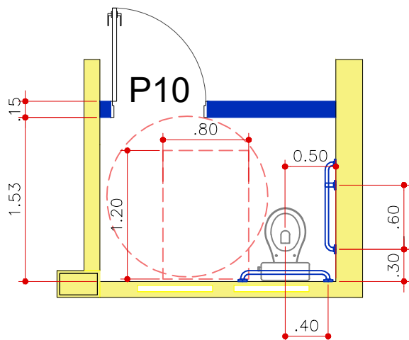
Planta baixa
