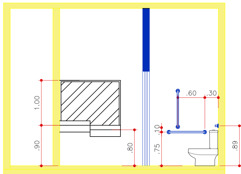
Elevação
