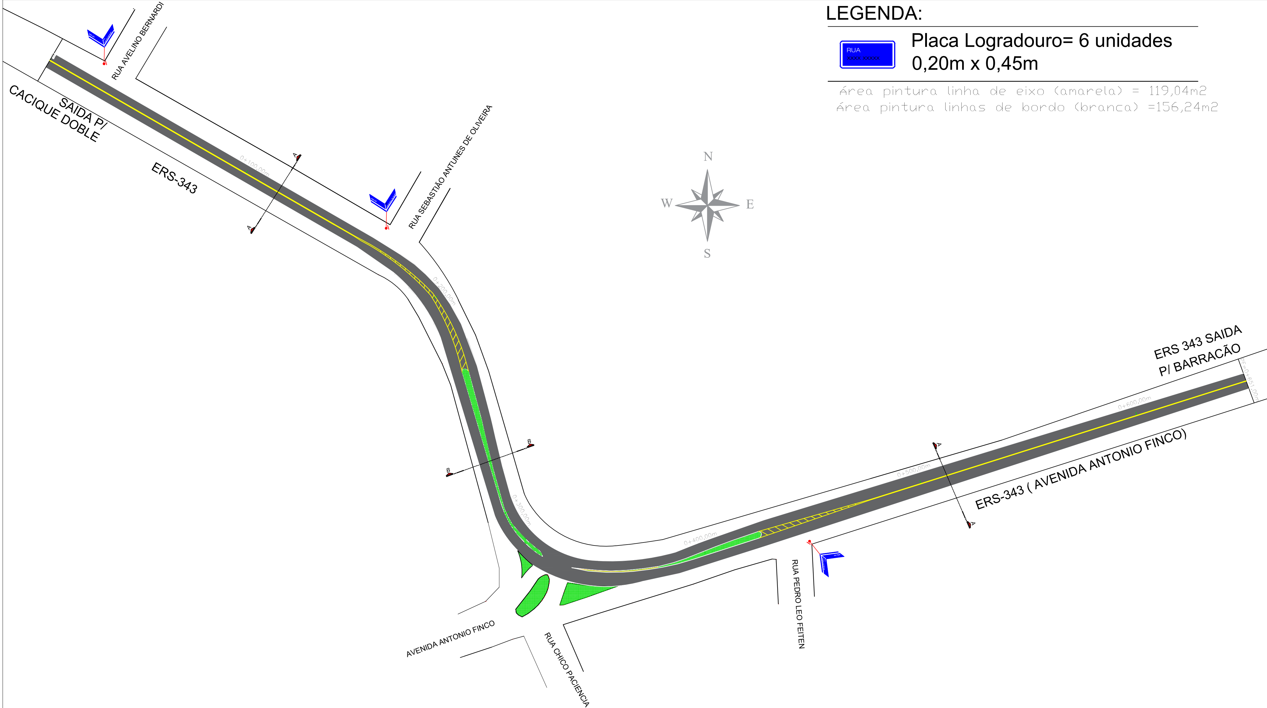
PLANTA SINALIZAÇÃO ESCALA 1:1.000
