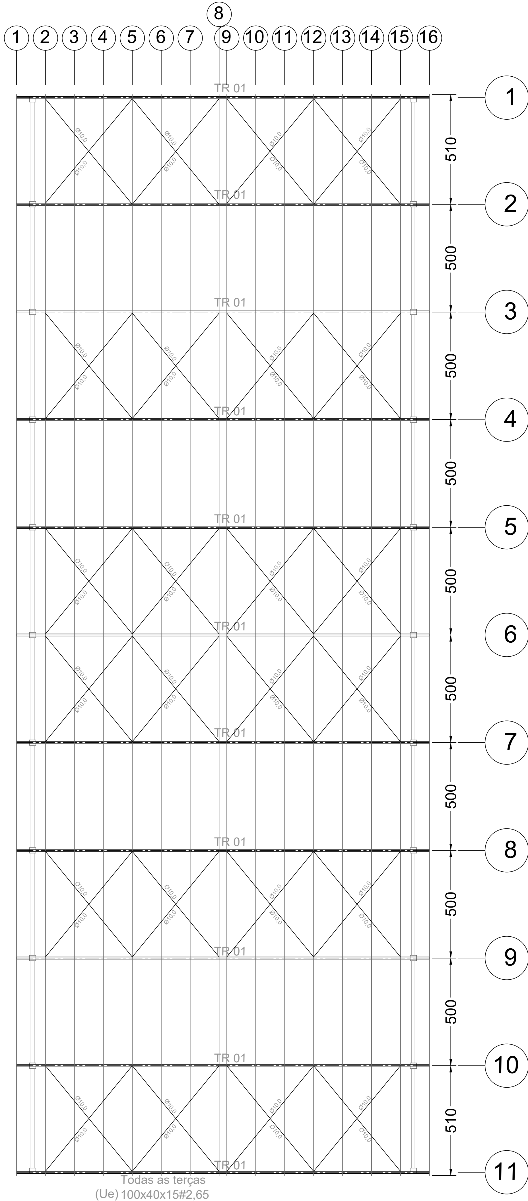
VISTA SUPERIOR - TERÇAS E TRAVAMENTOS ESC: 1/100
