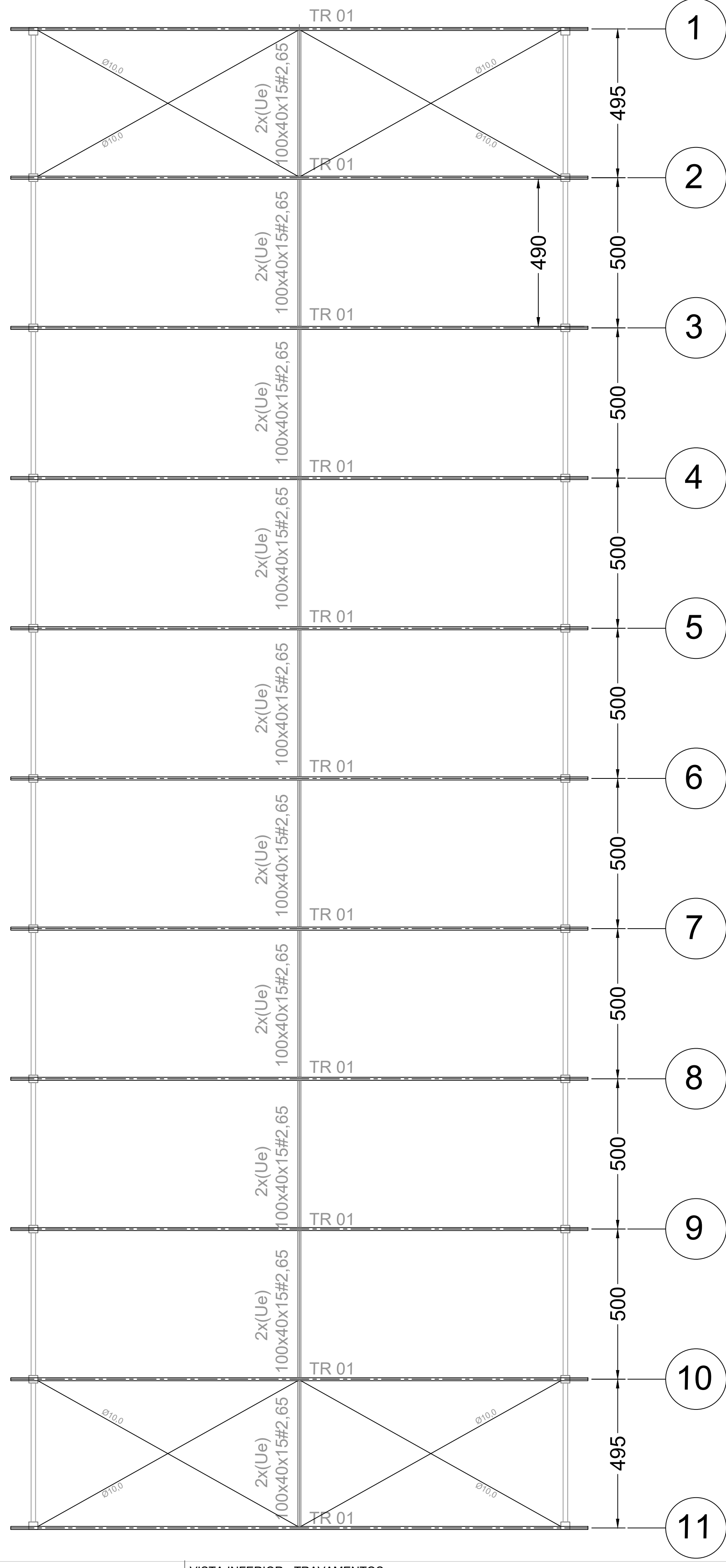
VISTA INFERIOR - TRAVAMENTOS ESC: 1/100
