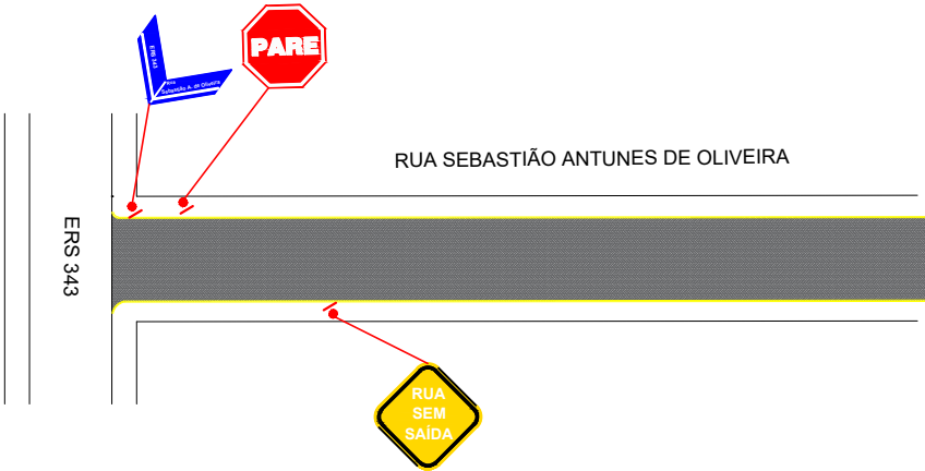
PLANTA SINALIZAÇÃO ESCALA 1:1.000
