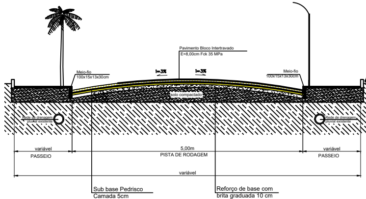
PERFIL VIÁRIO (SEM ESCALA) RUA MODESTO BÍSCARO
