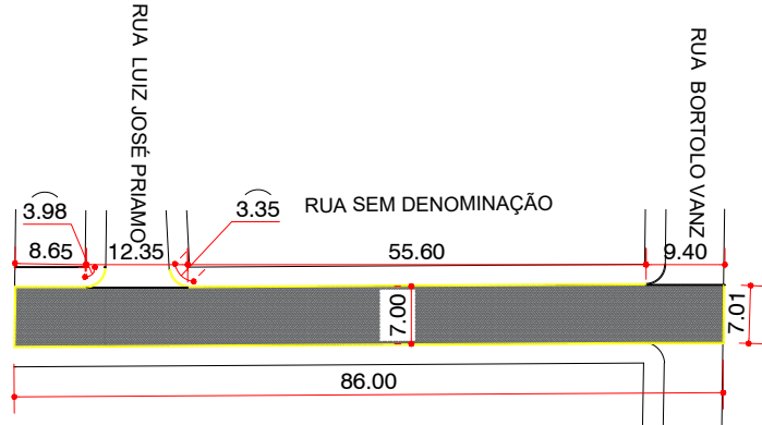
PLANTA PAVIMENTAÇÃO EM BLOCO INTERTRAVADO ESCALA 1:1.000
