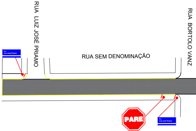
PLANTA SINALIZAÇÃO ESCALA 1:1.000
