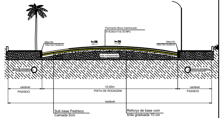
PERFIL VIÁRIO (SEM ESCALA) RUA SEBASTIÃO ANTUNES DE OLIVEIRA
