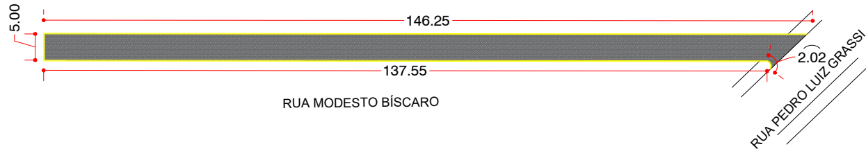
PLANTA PAVIMENTAÇÃO EM BLOCO INTERTRAVADO ESCALA 1:1.000
