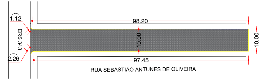
PLANTA PAVIMENTAÇÃO EM BLOCO INTERTRAVADO ESCALA 1:1.000
