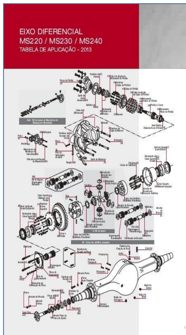
CONJUNTO DE DIFERENCIAL ILUSTRATIVO
