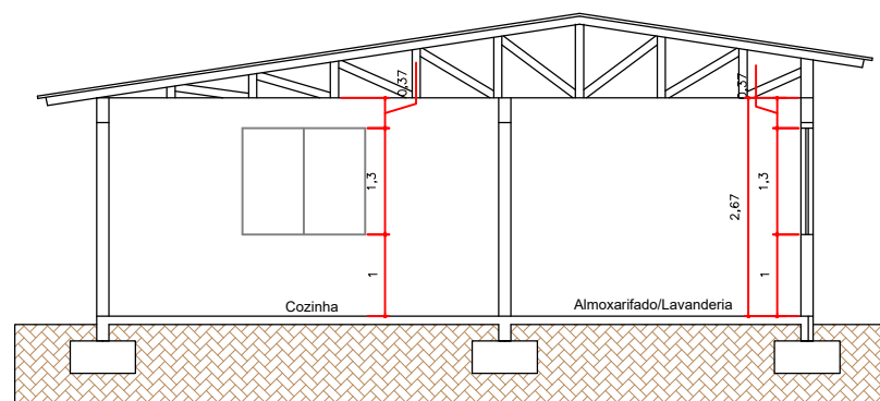
CORTE BB'
