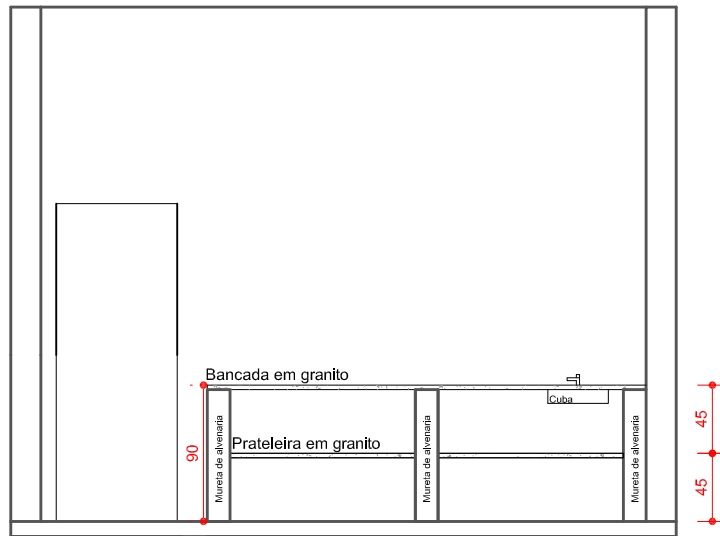
Vista bancada sala 1,2 e 3 Esc. 1:75
