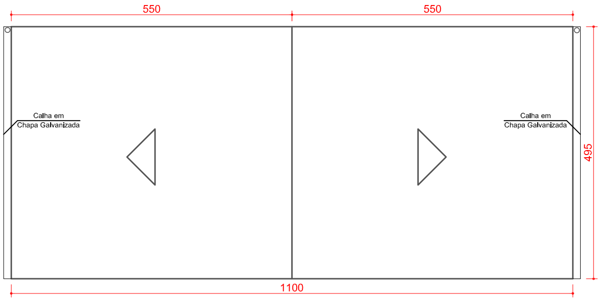
Vista toldo de lona Esc. 1:75
