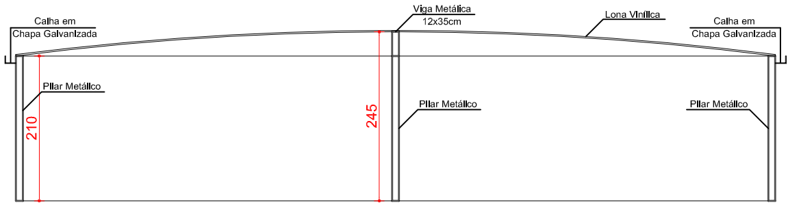
Corte toldo de lona Esc. 1:75
