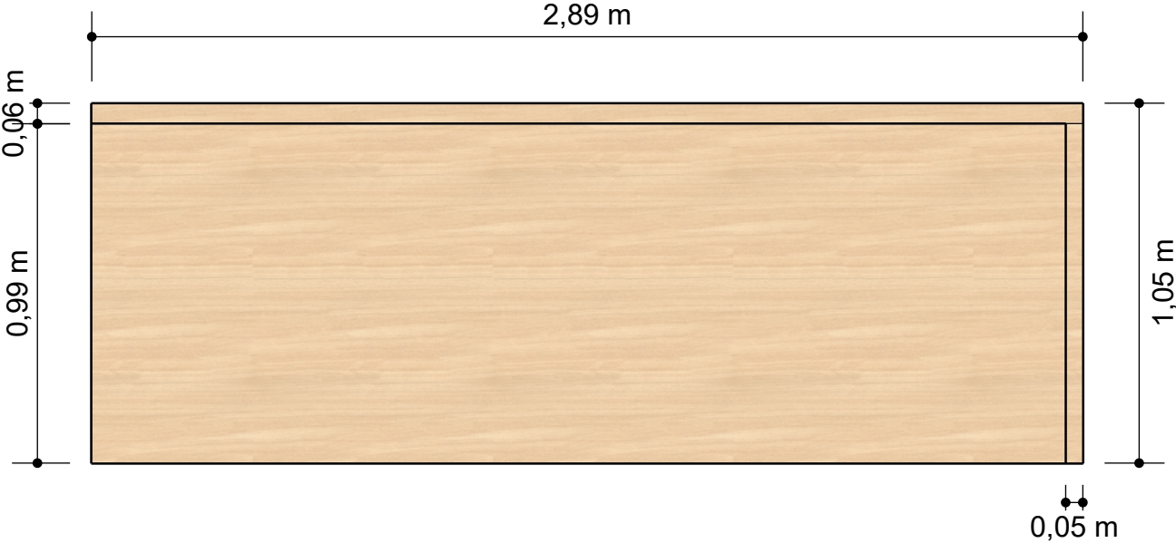
VISTA FRONTAL ESCALA 1:20
