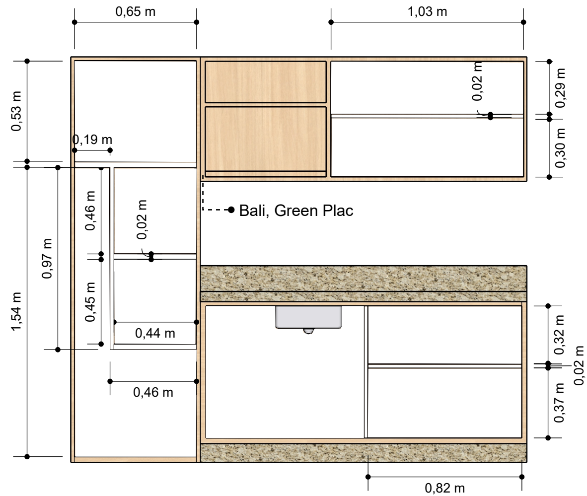
VISTA FRONTAL (PARTE INTERNA) ESCALA 1:20
