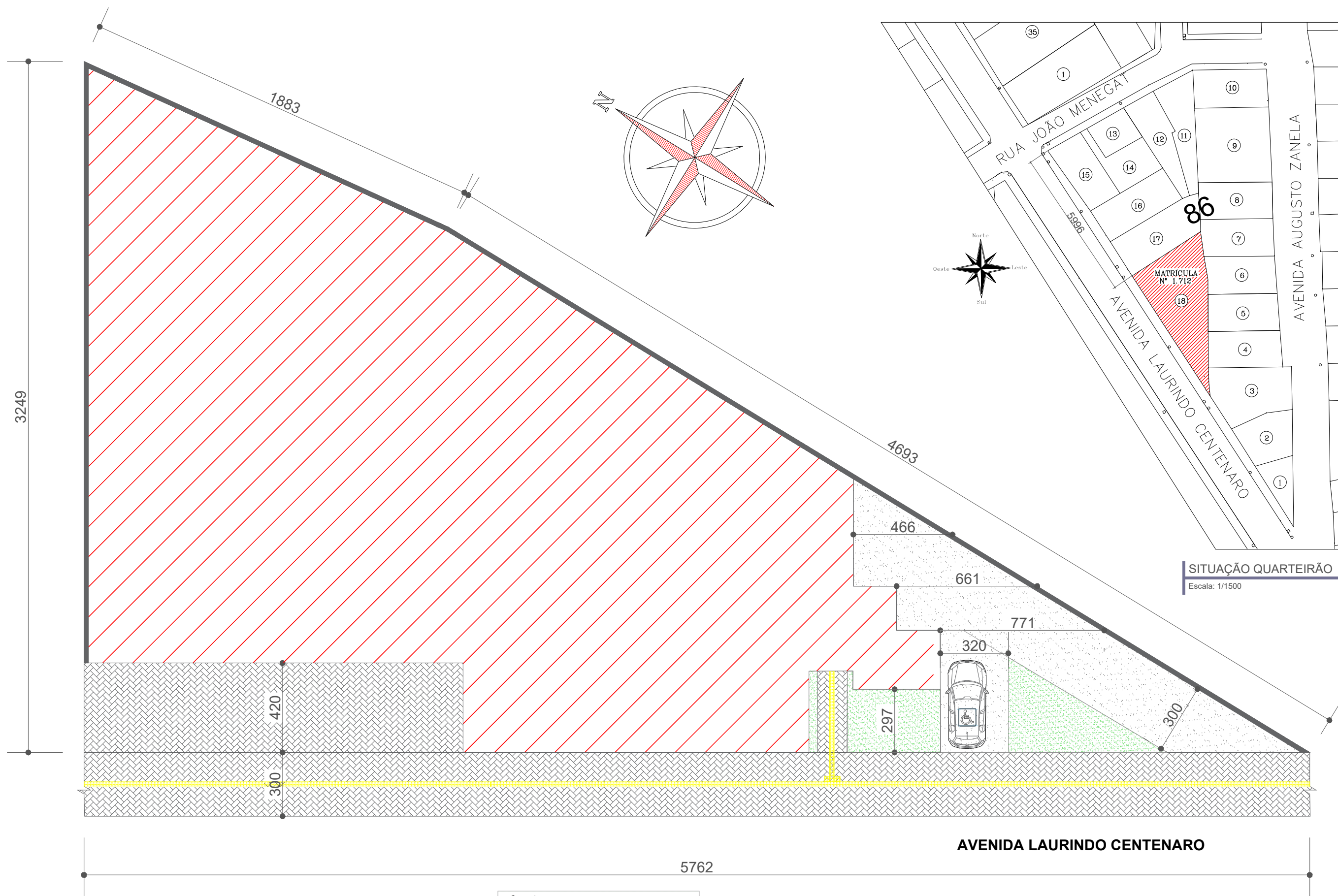
PLANTA DE LOCALIZAÇÃO Escala: 1/175
