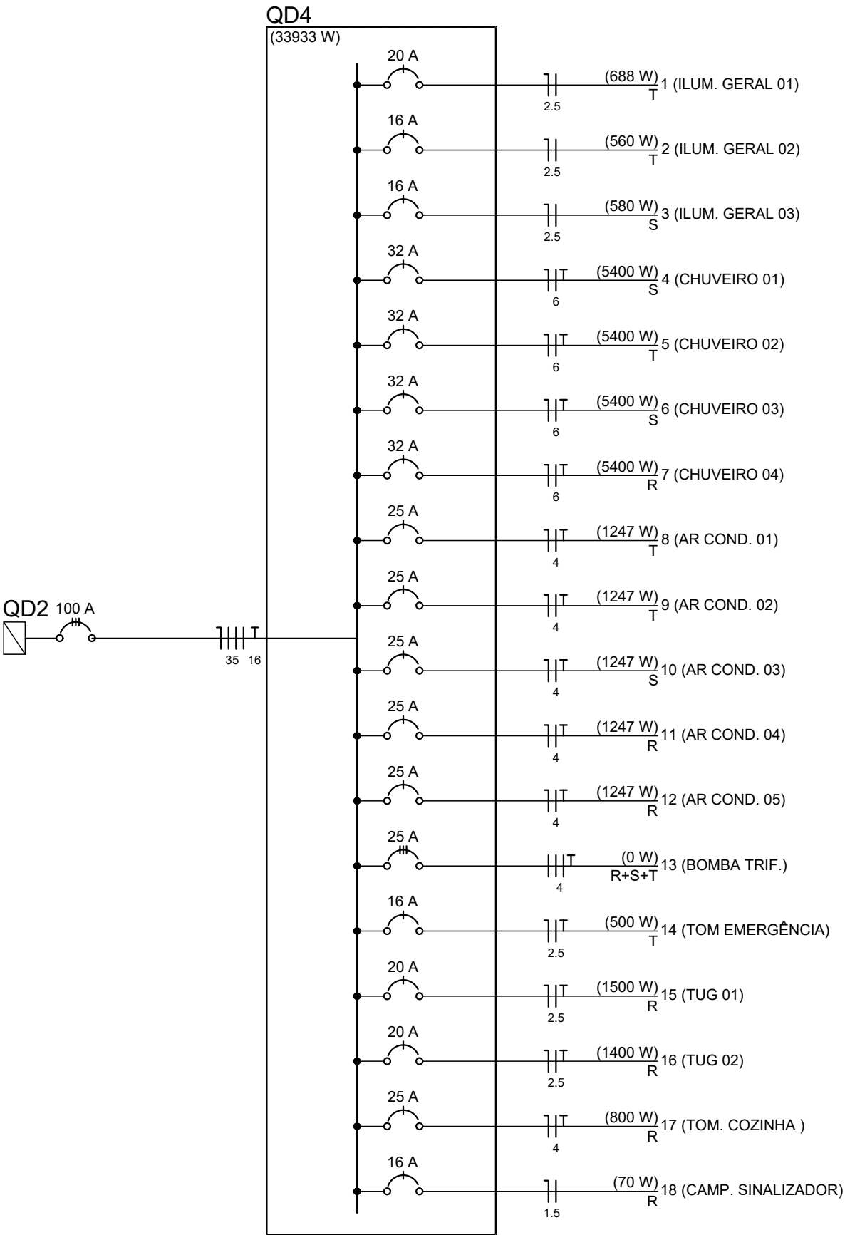
Quadro de Cargas (QD4)
